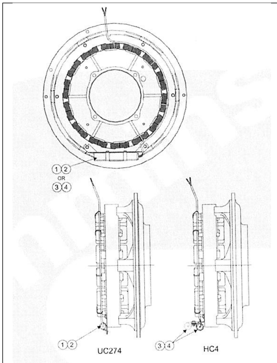
Рис.18 – Подогреватели генератора
