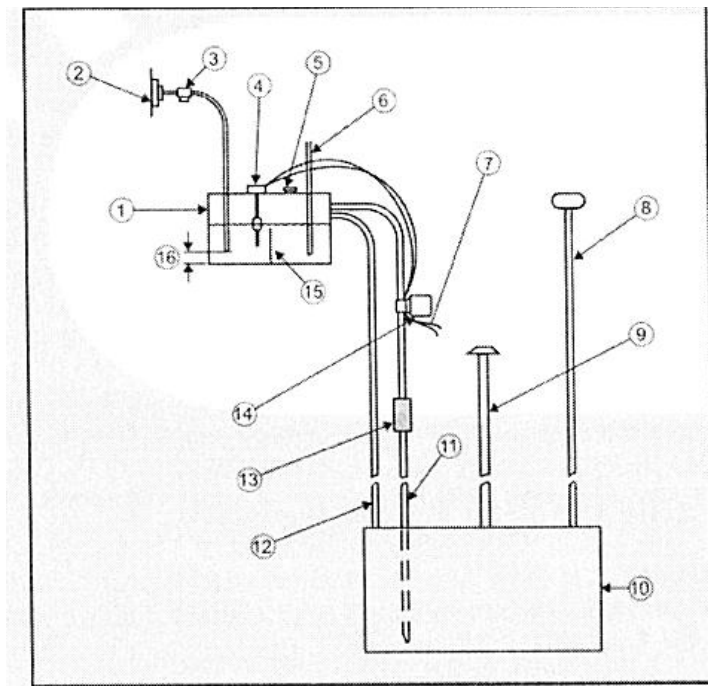
Рис. 7 Типовая конструкция топливной системы
