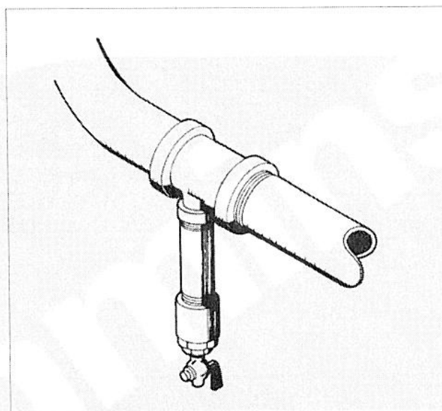
Рис. 9 – Ловушка для сбора конденсата
