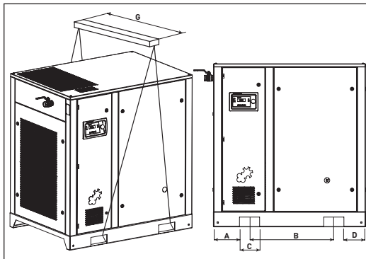
Bild 3.1 Heben und Transportieren DV30–55
