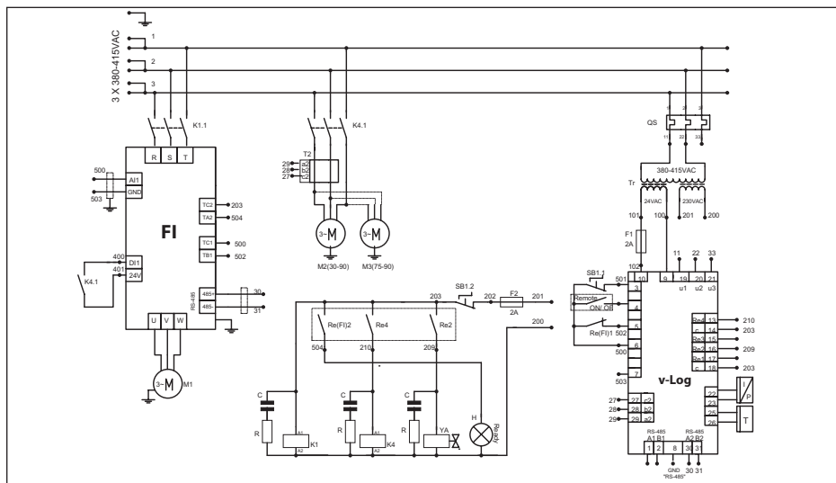
Рис. 2.6 Схема электрическая DV30-55
