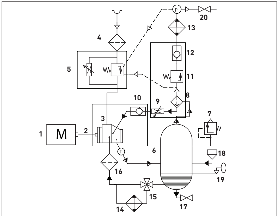
Bild 2.3 Ablaufdiagramm DV30-55
