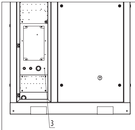
Рис. 3.6.2 Подключение к электропитанию
