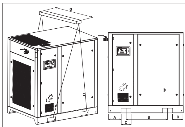
Рис. 3.1 Схема для такелажных работ DV30-55
