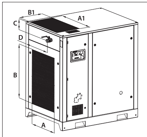
Bild 3.3 Einbauabmessungen DV30-55
