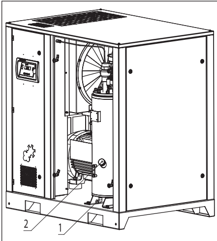
Bild 5.7 Austausch des Luft/Öl-Separator
