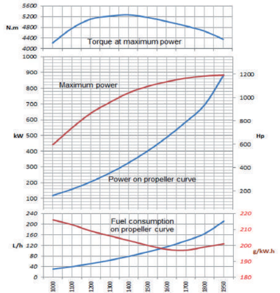
P2 - 883 kW - 1200 hp @1950 rpm
